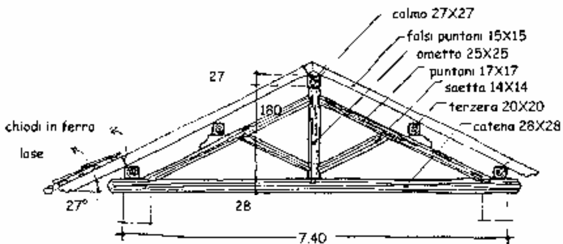
capriata esistente
