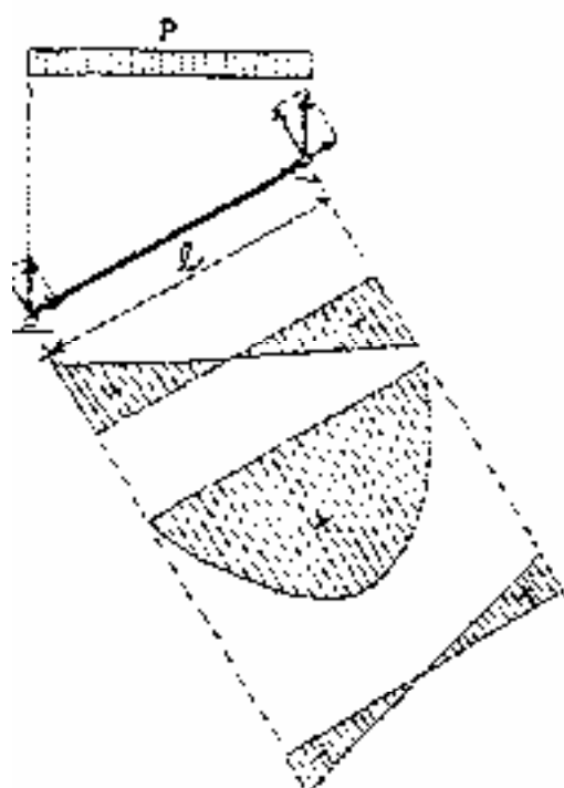
sistema stativo falso puntone
