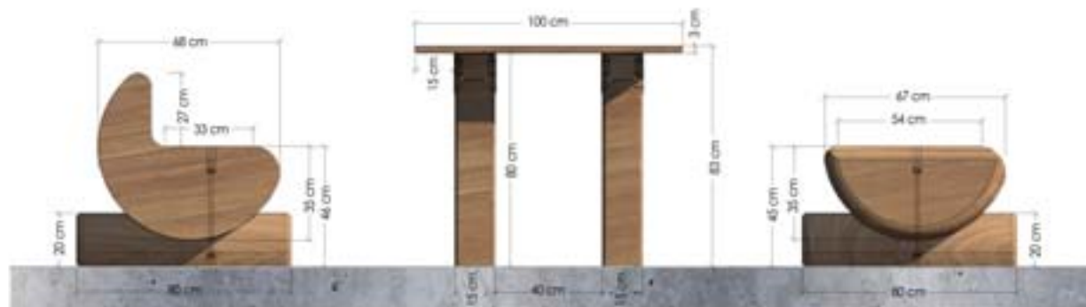
Prospetto laterale delle panche e del tavolo
