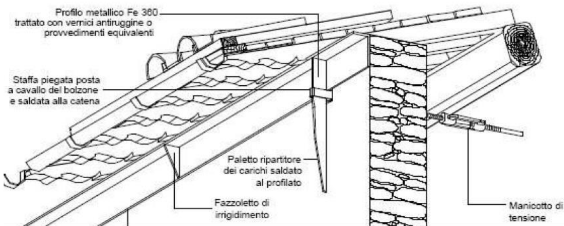
Esempio di cordolo in acciaio
