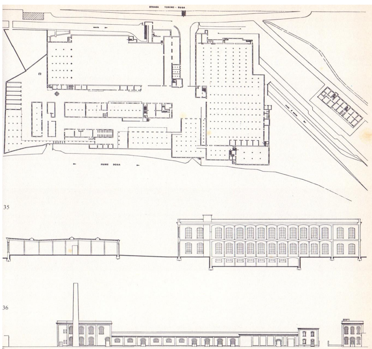
Schema d'impianto del Cottonificio Wild & Abegg, Chianocco
